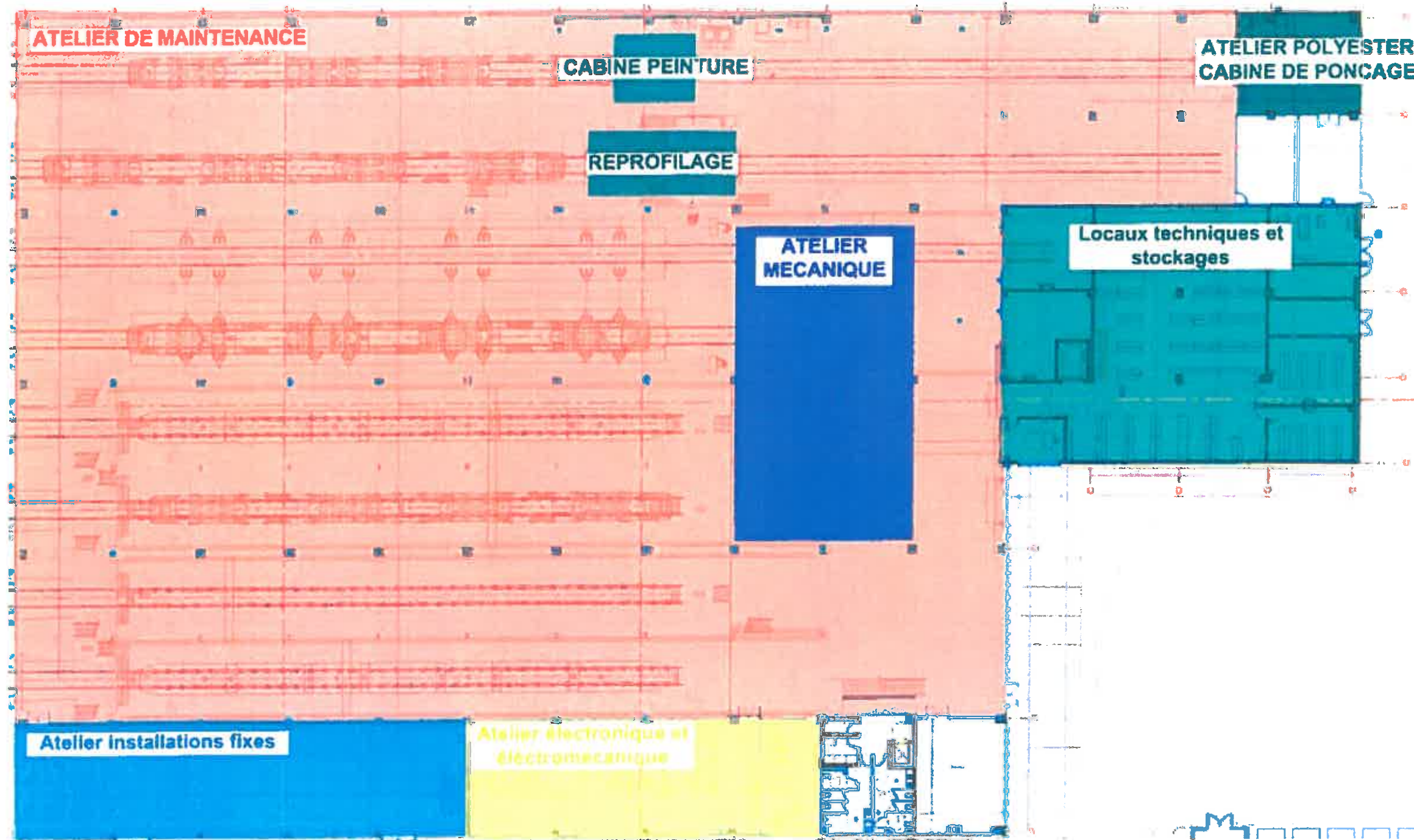
Figure 2 : Plan d'implantation des différents activités dans le bâtiment de maintenance
